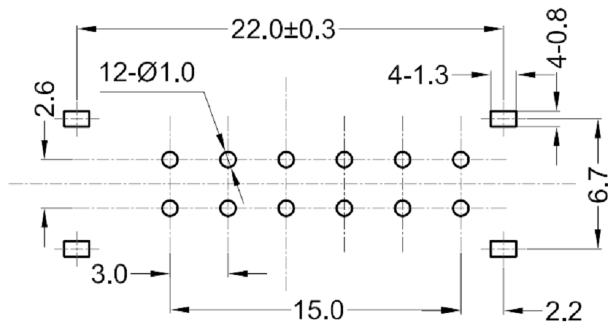
P.C.B LAYOUT
